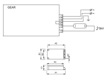
Technische Daten Philips HID-PV 100 /S SDW-TG 220-240V 50/60Hz für 100W
